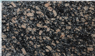
Гранит КОРНИНСКИЙ
