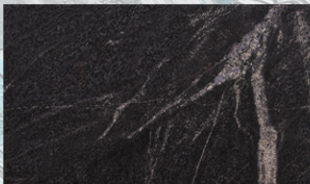
Гранит РАХНЫ-ПОЛЕВКИЙ
