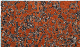
Гранит КАПУСТИНСКИЙ
