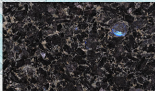
Лабр. ОСНЫКОВСКИЙ
