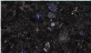
Лабр. ОЛЕГОВСКИЙ
