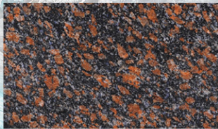
Гранит БРУСИЛОВСКИЙ
