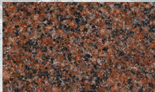
Гранит КОРЕЦКИЙ
